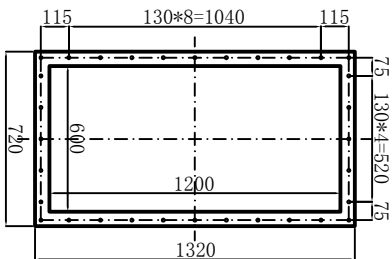
进出口风口尺寸
