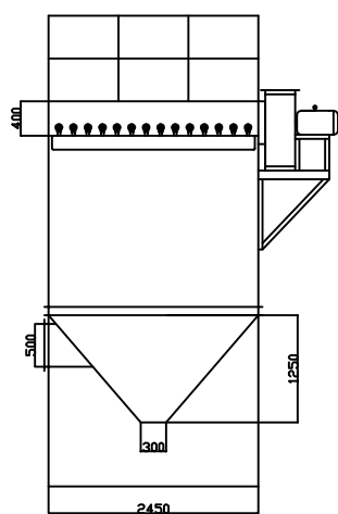
mc-140 袋裝全器圖
