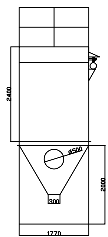
mc-140 袋裝全器圖
