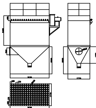
mc-180 机械全图
