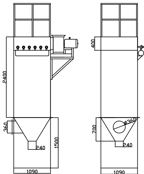
mc-36 袋除尘器图
